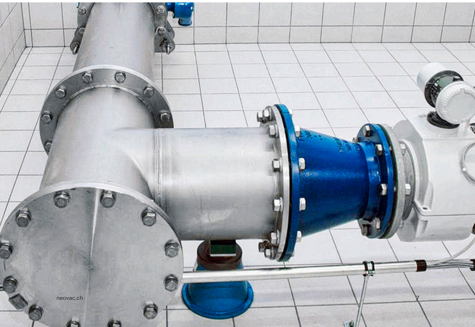
Condotte di erogatori a sorgente guidate tramite impianto UV ↑
