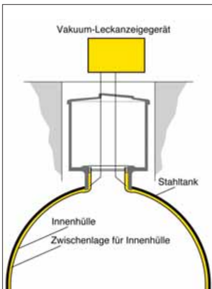
Prinzipschema
