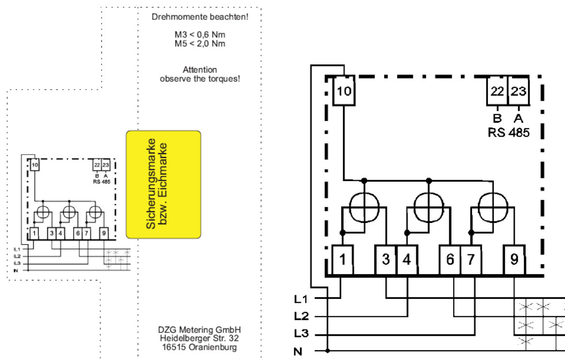
Fig. 4: Schaltbild
