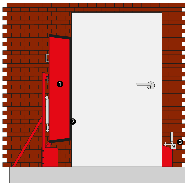
Paratia per acqua antincendio automatica, al di fuori dell'intradosso
