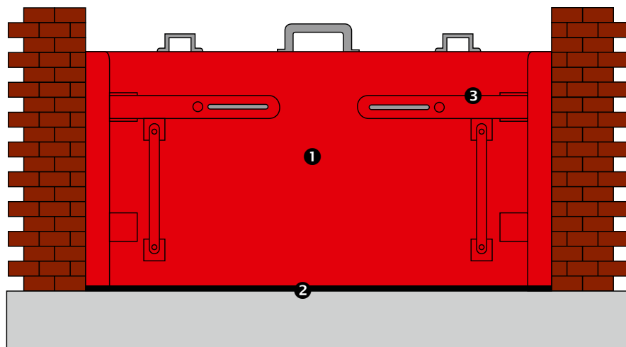
Paratia per acqua antincendio manuale, montaggio all'interno dell'intradosso
